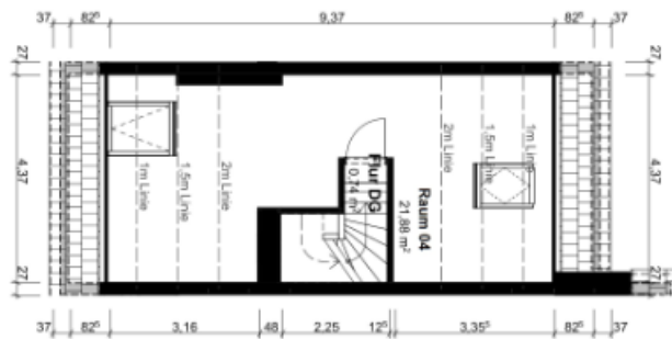
Dachgeschoss
